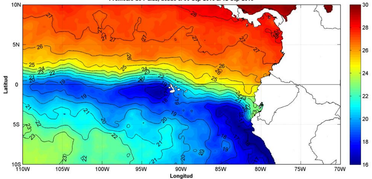
ANÁLISIS DE TSM 4 km, UKMO/INOCAR (grados Celsius) Promedio de 7 días, desde el 06-Sep-2010 al 12-Sep-2010
