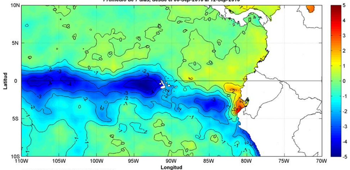
ANÁLISIS DE ANOMALÍA DE TSM 4 km, UKMO/INOCAR (grados Celsius) Promedio de 7 días, desde el 06-Sep-2010 al 12-Sep-2010
